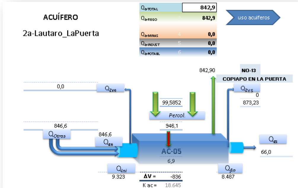
Figura 11-2: ESQUEMA BALANCE HIDRICO ACUIFEROS 05
